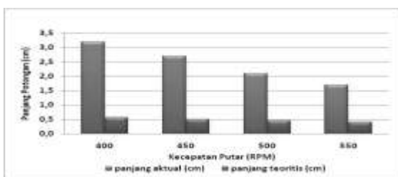
Gambar 9. Panjang rata-rata pemotongan serasah tebu
